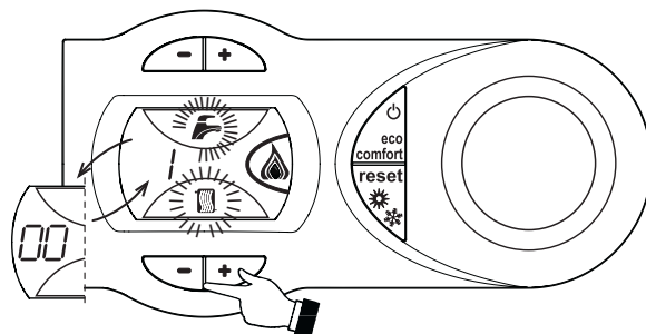
fig. 15 - Modalità TEST (potenza riscaldamento = 100%)
