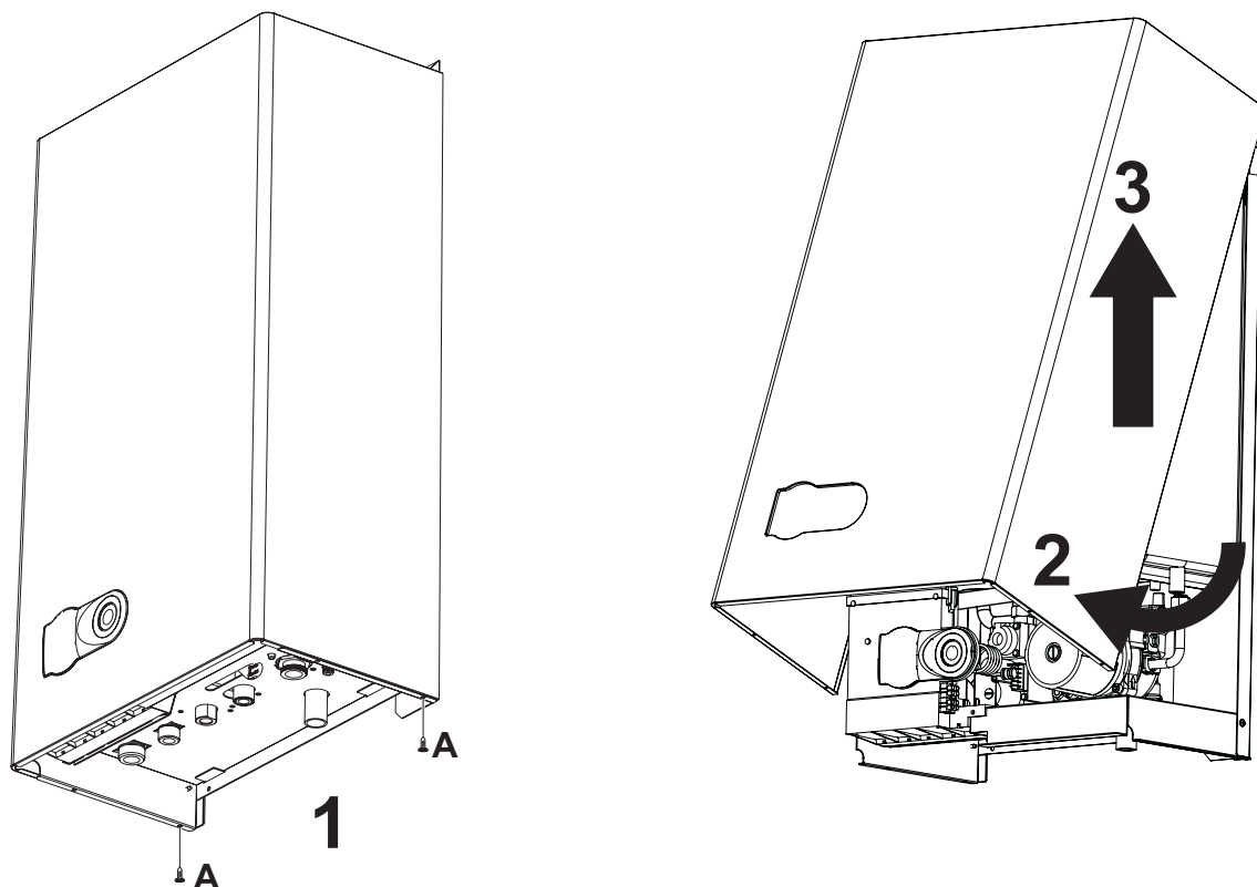
fig. 17 - Apertura mantello
