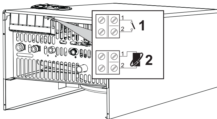
fig. 14 - Accesso alla morsettiera
