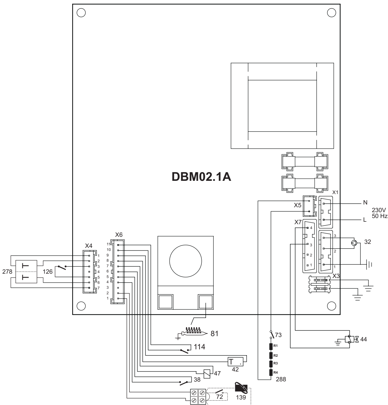
fig. 21 - Schema elettrico
