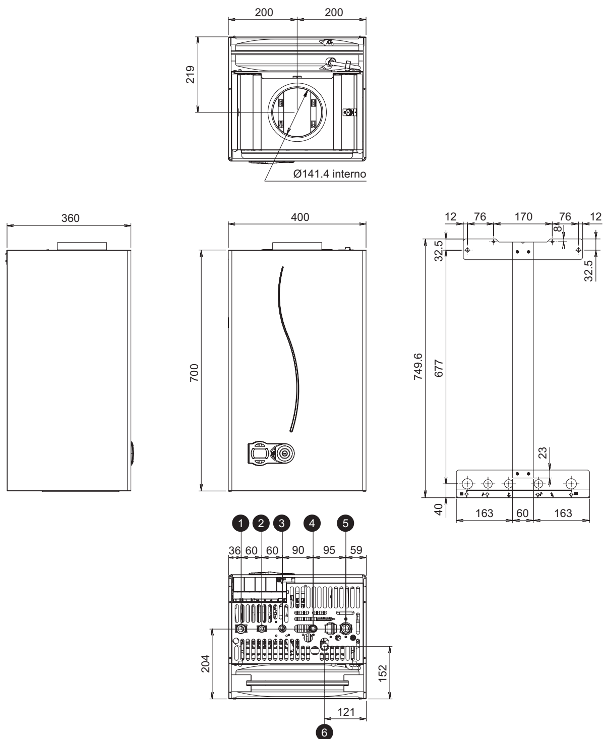
fig. 18 - Dimensioni e attacchi
