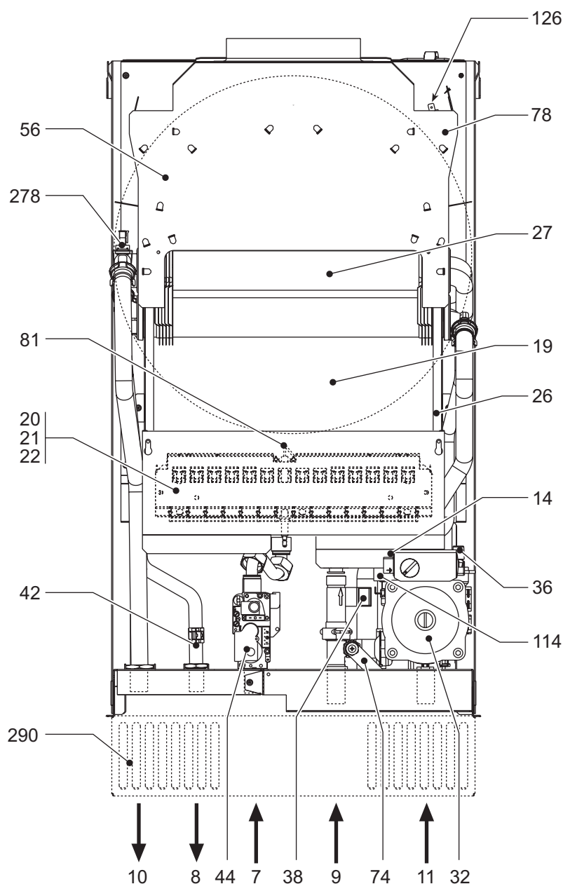
fig. 19 - Vista generale
