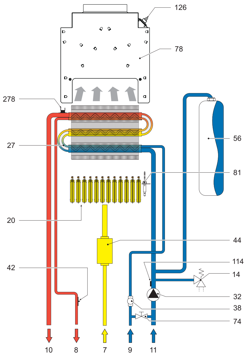
fig. 20 - Circuito idraulico
